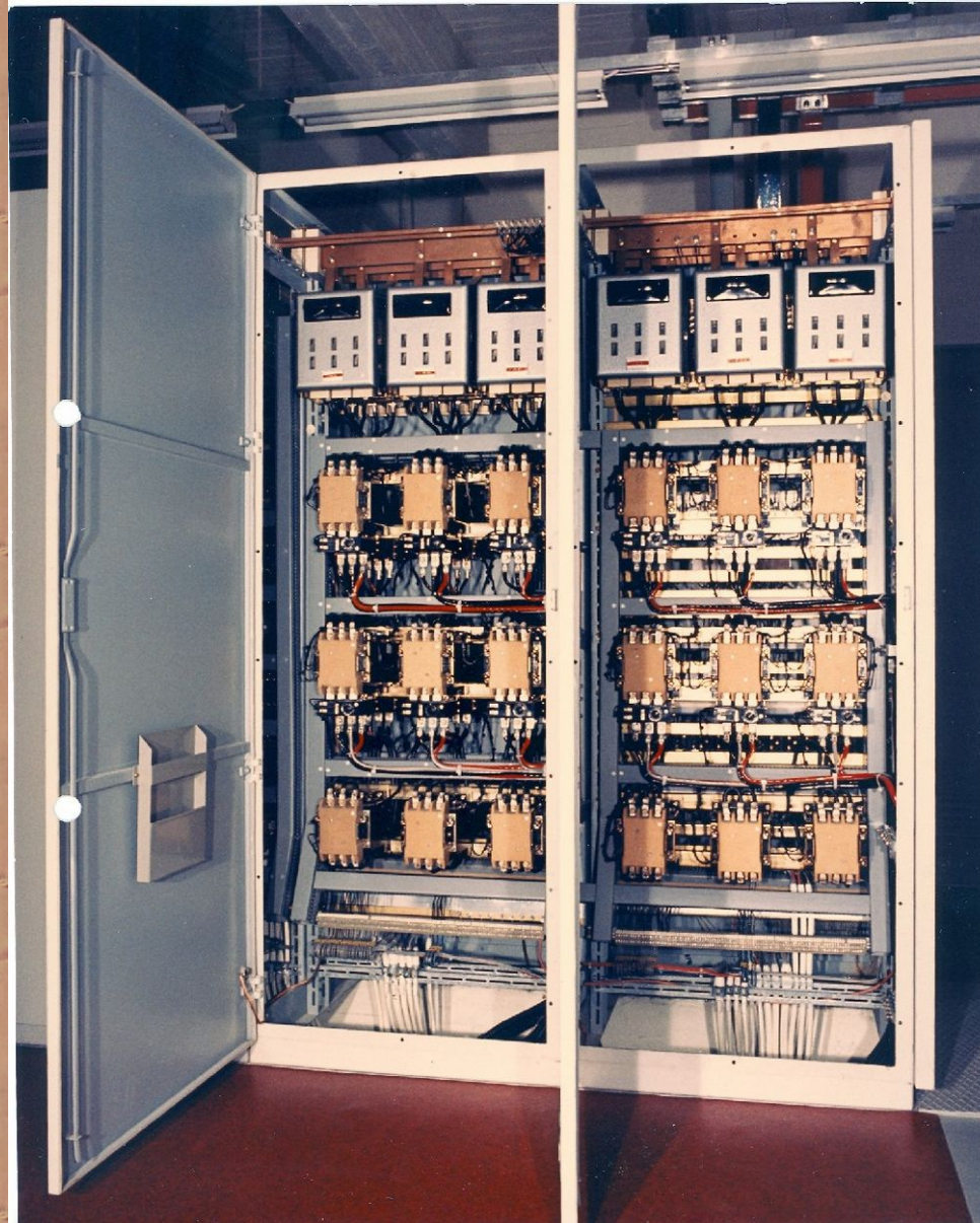
Armoire de distribution BT Schaltschrank
